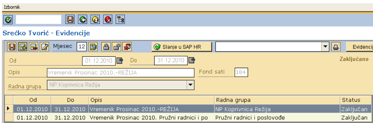
Slika 62: Evidencije
