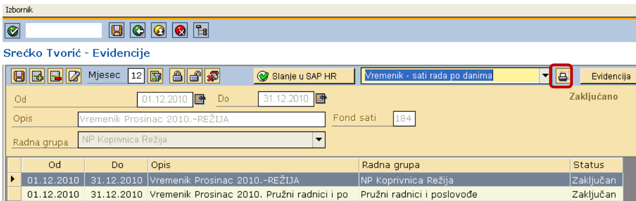
Slika 64: Evidencije
