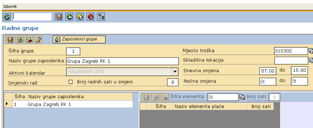
Slika 24:radne grupe
