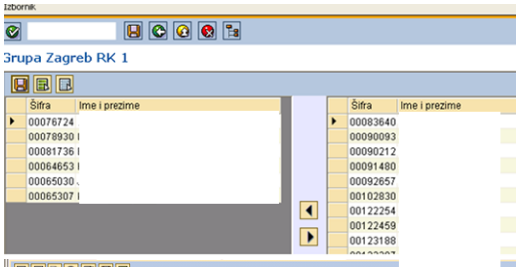
Slika 39: lista zaposlenika
