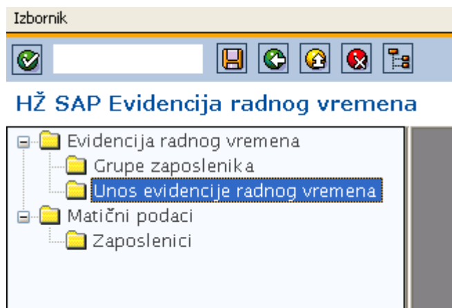
Slika 61:izbornik
