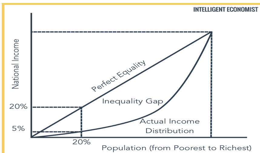
Slika 1. Lorenzova krivulja
