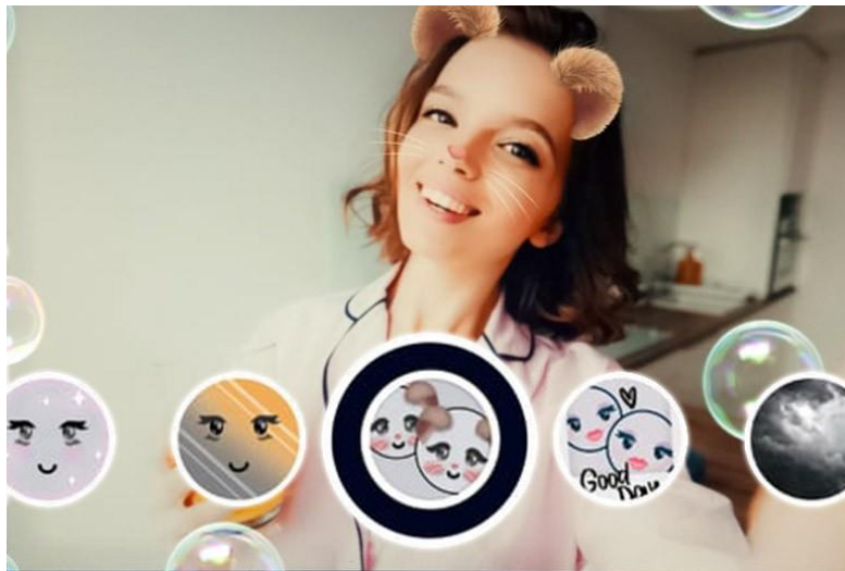
Slika 11. Snapchat aplikacija
