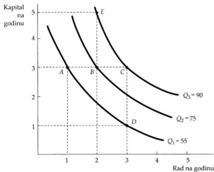
Graf 4.4.1. Proizvodnja s dva varijabilna faktora
