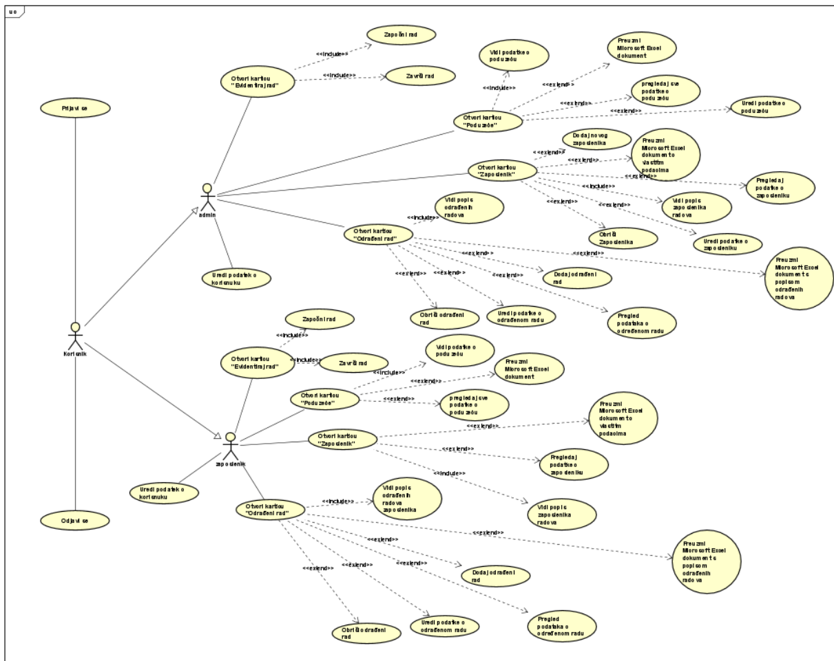
Slika 13. Dijagram slučajeva korištenja programske aplikacije "Evidencija_radnog_vremena_zaposlenika"
