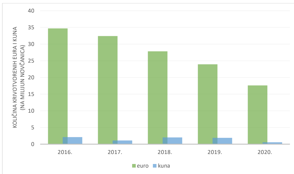
Grafikon 7. Količina krivotvorenih kuna i eura na milijun novčanica u razdoblju od 2016. do 2020. godine
