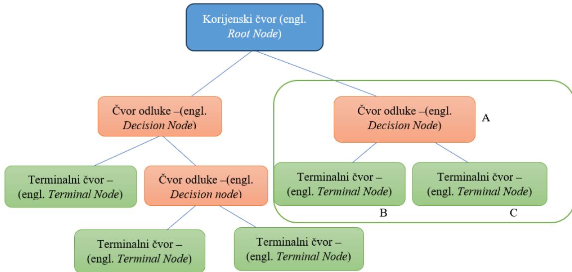
Slika 16. Stablo odlučivanja
