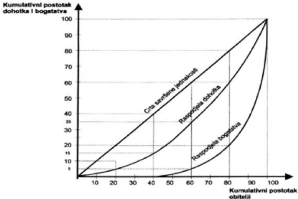
Slika 6. Lorenzova krivulja
