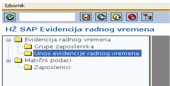
Slika 40: izbornik
