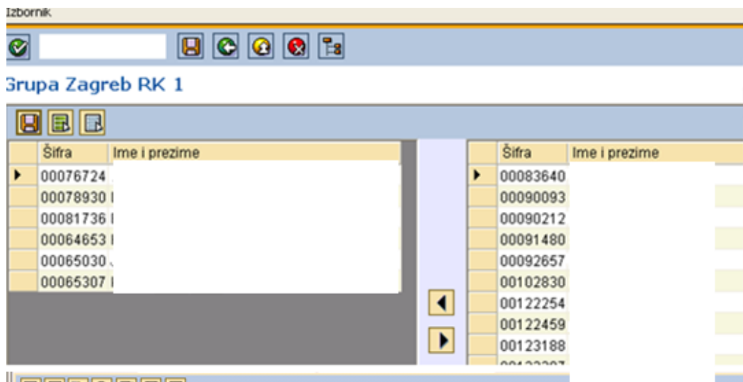
Slika 39: lista zaposlenika
