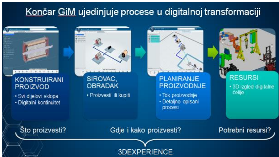
Slika 2. Prikaz kako digitalna transformacija može unaprijediti proces proizvodnje generatora
