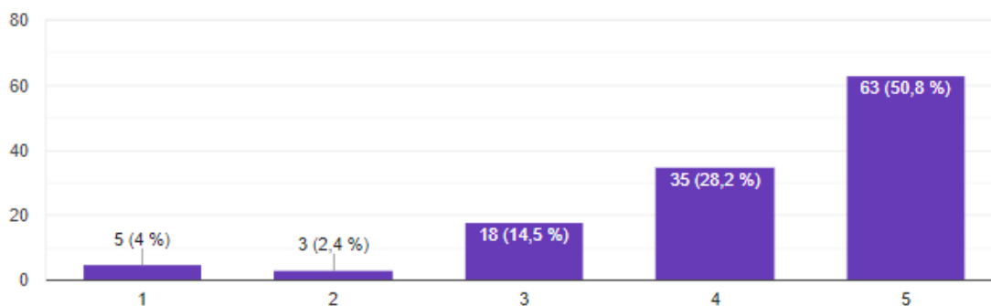
Slika 23. Važnost oglašavanja na društvenim mrežama
