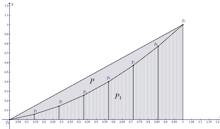
Slika 1. Lorenzova krivulja
