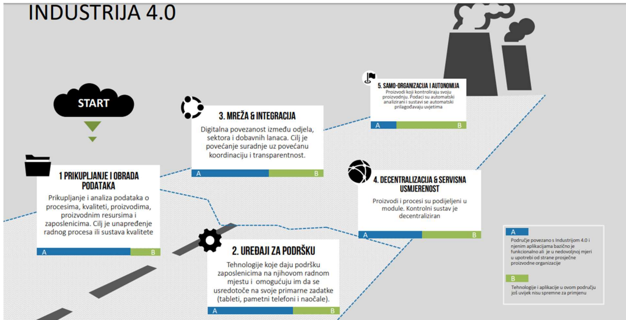
Slika 12: Industrija 4.0
