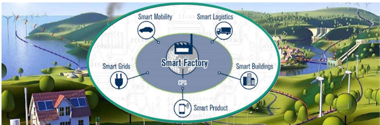
Slika 13: Industrija 4.0
